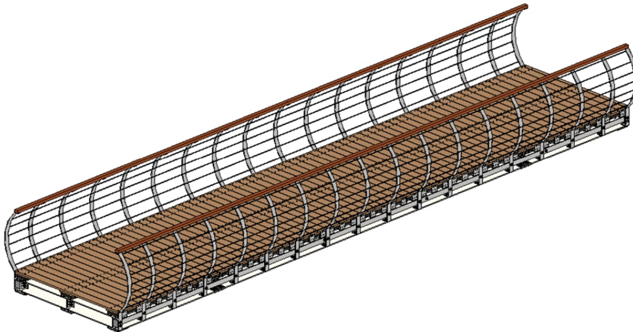
Figuur 49: De CMD-brug
