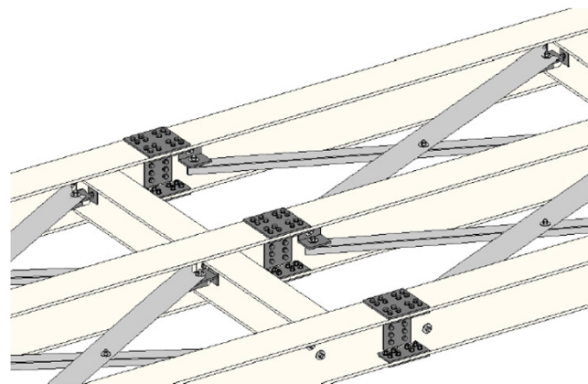
Figuur 51: Detail van stalen draagstructuur van het definitieve ontwerp
