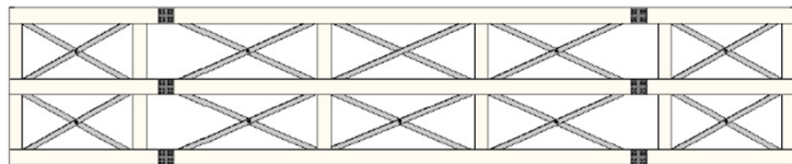
Figuur 50: Stalen draagstructuur van het definitieve ontwerp
