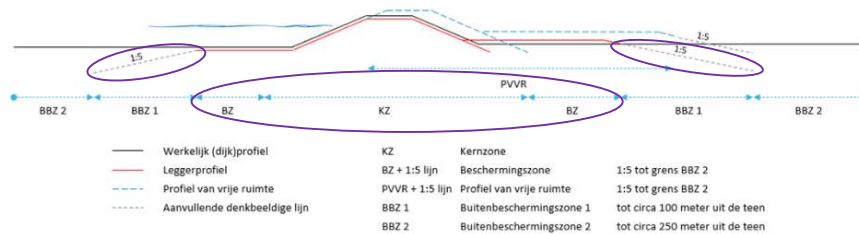
Leggerprofiel dijk
