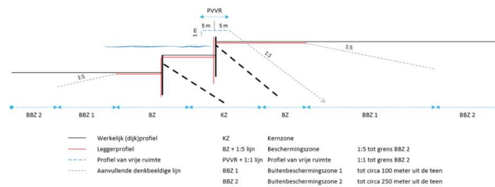
Leggerprofiel langsconstructie
