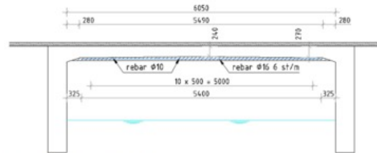
Figuur 5: langsdoorsnede met re-bar
